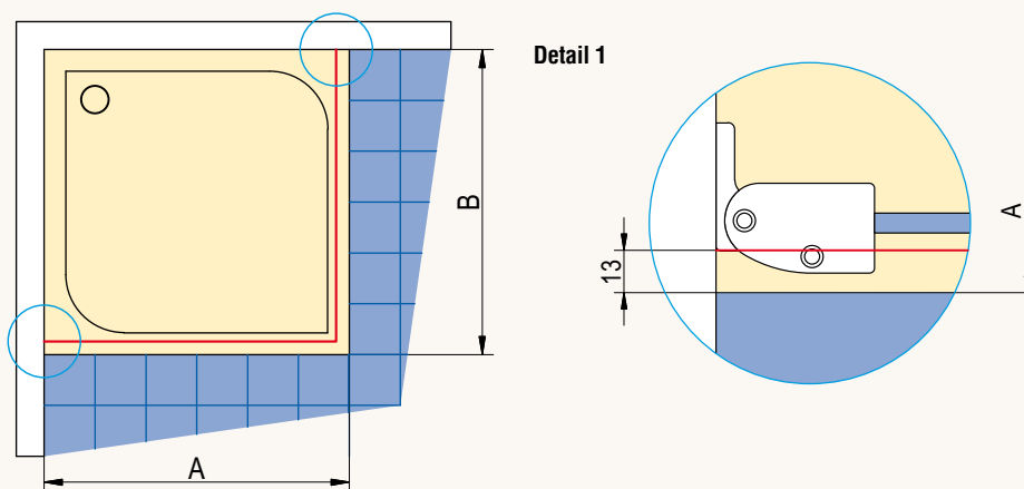
Instalační rozměr vaničky pro zástěnu standardních rozměrů
